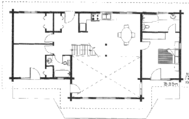
Grundrissplan Erdgeschoss
