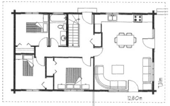
Grundrissplan Erdgeschoss
