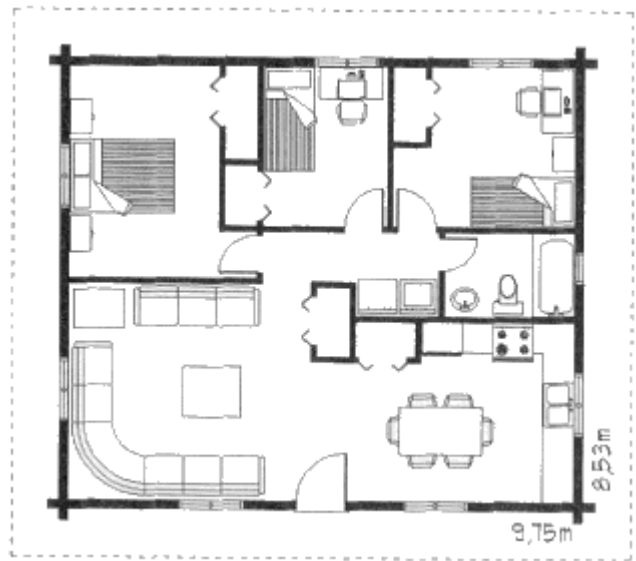
Grundrissplan Moose -2-
