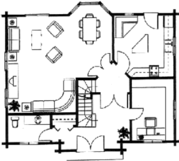
Grundrissplan Erdgeschoss
