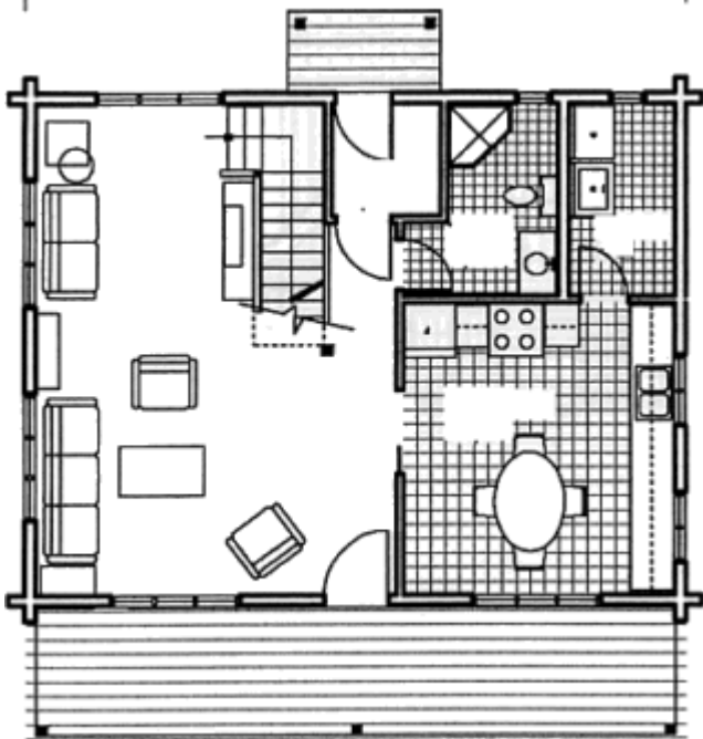
Grundrissplan Erdgeschoss
