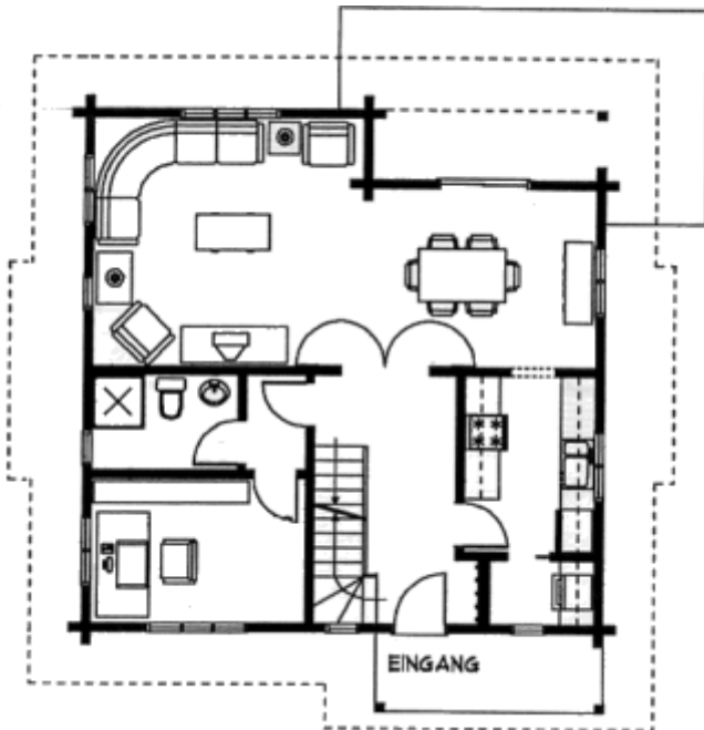
Grundrissplan Erdgeschoss
