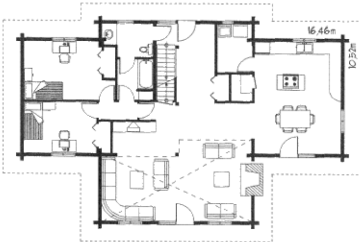
Grundrissplan Erdgeschoss
