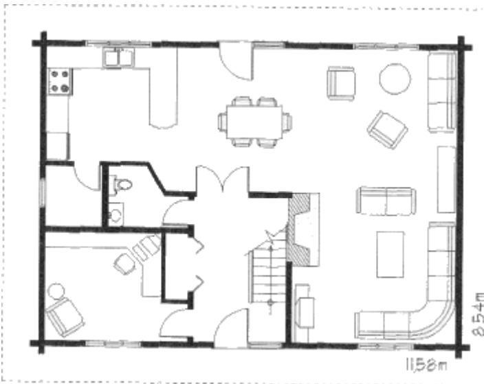
Grundrissplan Erdgeschoss
