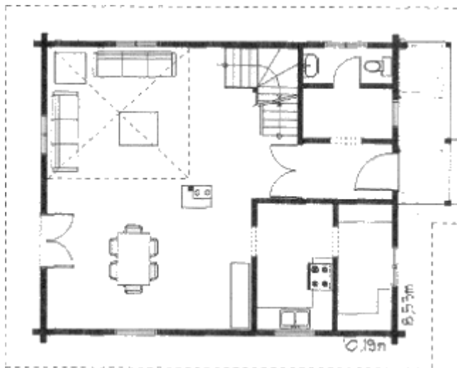
Grundrissplan Erdgeschoss
