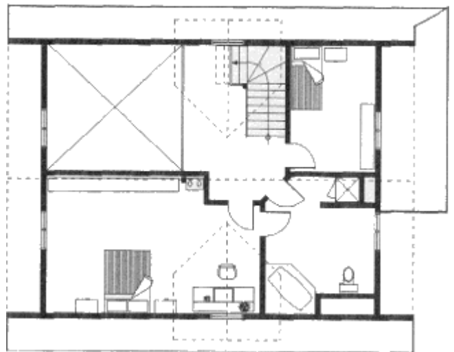
Grundrissplan Dachgeschoss
