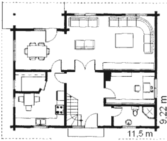
Grundrissplan Erdgeschoss
