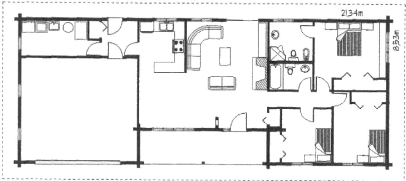
Grundrissplan Erdgeschoss
