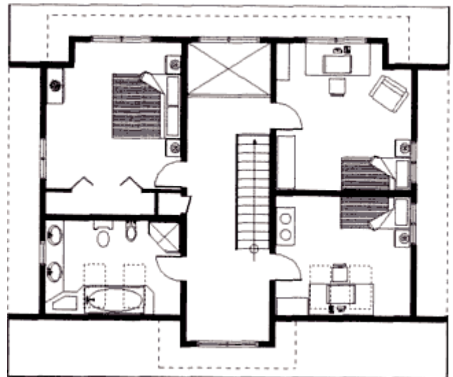
Grundrissplan Obergeschoss
