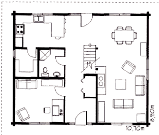
Grundrissplan Erdgeschoss
